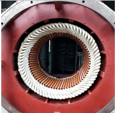
SỬA CHỮA QUẤN STATOR MÁY PHÁT 1250KVA – 6,6KV NHÀ MÁY THỦY ĐIỆN BÙ CÀ MAU REPAIR OF STATOR WINDING GENERATOR 1250KVA – 6.6KV BU CA MAU HYDROPOWER PLANT
